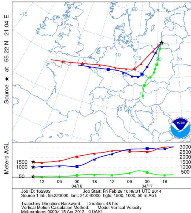
4 pav. Oro masių pernašos atgalinės trajektorijos, 2013 metų balandžio 18 d.
