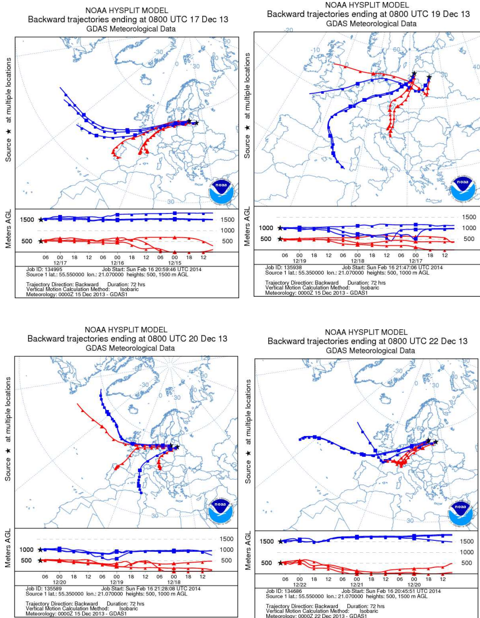
9 pav. Oro masių judėjimo 72 val. atgalinės trajektorijos 2013 m. gruodžio mėn. 17, 19, 20 ir 22 d. į IM stotis ir Preilą. Šaltinis: http://ready.arl.noaa.gov/HYSPLIT_traj.php
