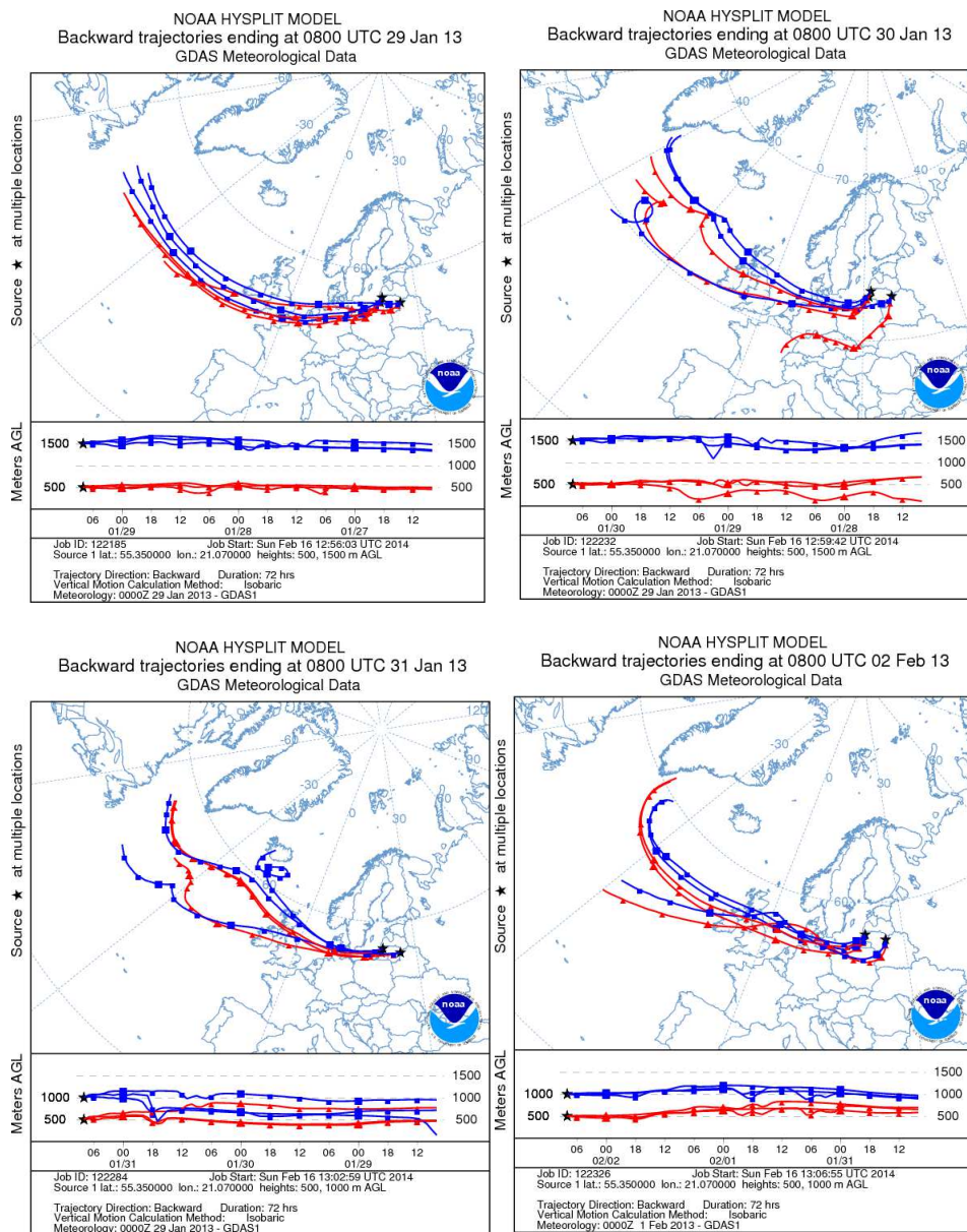
7 pav. Oro masių judėjimo 72 val. atgalinės trajektorijos 2013 m. sausio mėn. 29 – vasario 2 d. į IM stotis ir Preilą. Šaltinis: http://ready.arl.noaa.gov/HYSPLIT_traj.php
